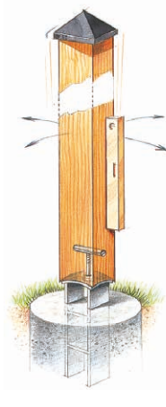
Zanche ad H con bullone
