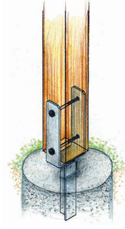
Zanche ad U da annegare nel cemento
