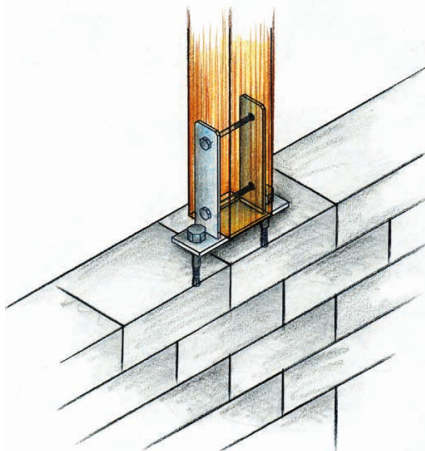
Pedistallo per fissaggio con bulloni su pavimentazione o muri
