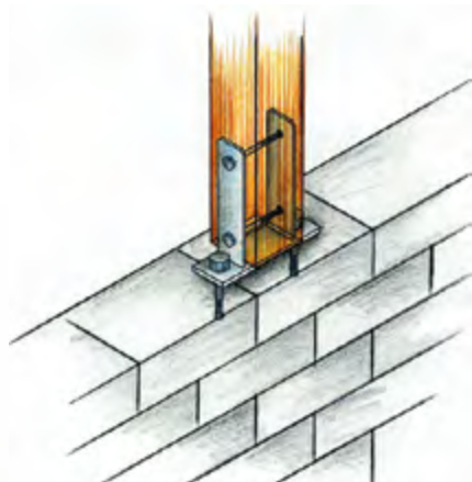
Piedistallo per fissaggio con bulloni su pavimentazione o muri
